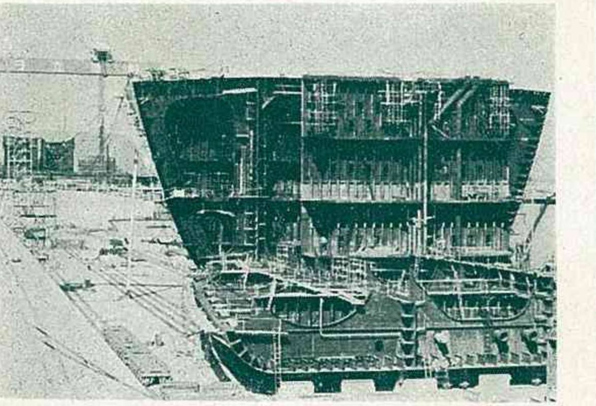
船首部と船尾部のドッキングも間近、23万トンタンカー (日立造船有明工場で)
