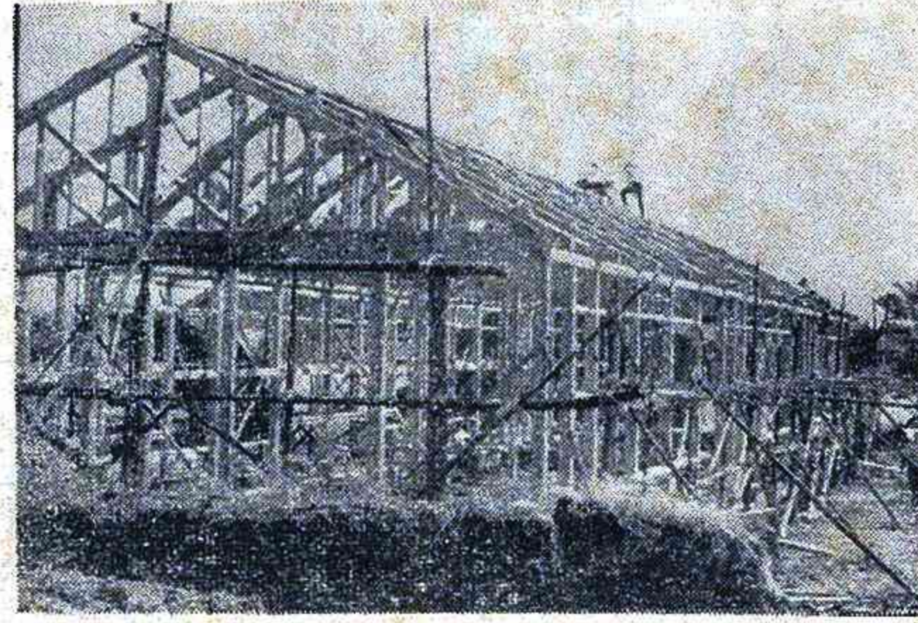
写真は 長洲中学校増築現場
