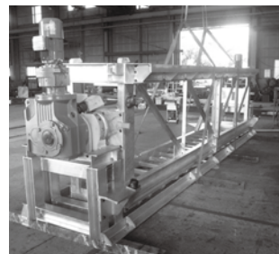
製氷工場向け脱氷機
