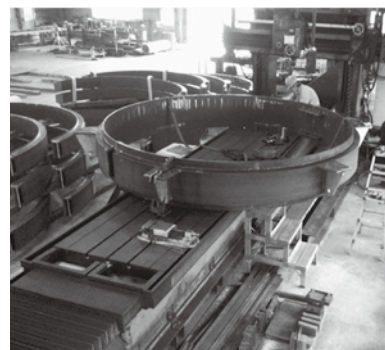
火力発電所の煙突固定点リング製作風景
