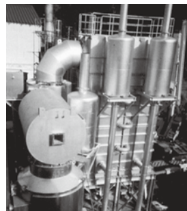
産業廃棄物の焼却炉全景
